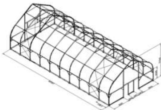
Схема каркаса ангара серии АП
