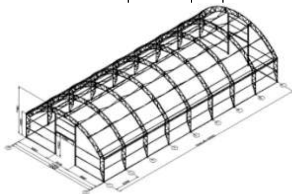
Схема каркаса ангара серии В
